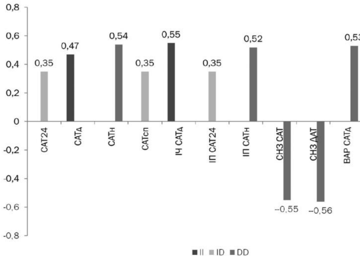
Рисунок 1. Кореляційний взаємозв'язок між показниками добової величини ІММЛШ/зріст 2,7
